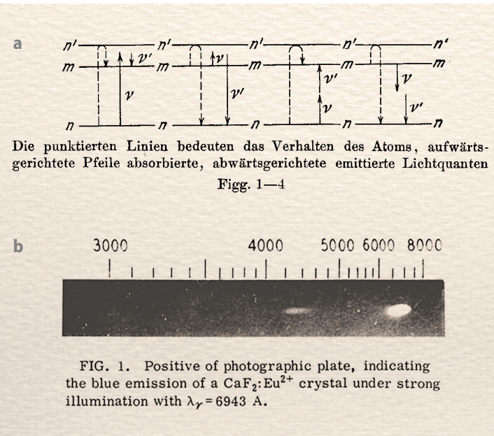
Abb. 2 Maria Goeppert Mayers Übergangsschema bei Zwei-Photonen-Prozessen (a). Der linke schwache Punkt zeigt die von Wolfgang Kaiser und Charles Garrett im Jahr 1961 beobachtete Fluoreszenz bei 425 nm, induziert durch einen Zwei-Photonen-Absorptionsprozess (b).
