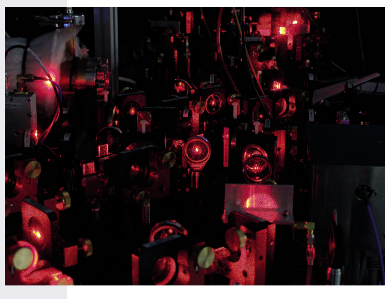
Bild oben links Geschwindigkeitsverteilung kalter bosonischer Gase beim Kühlen bis zur Bose-Einstein-Kondensation. Die Temperatur sinkt von links (thermische Atomwolke) nach rechts (Bose-Einstein-Kondensat).
